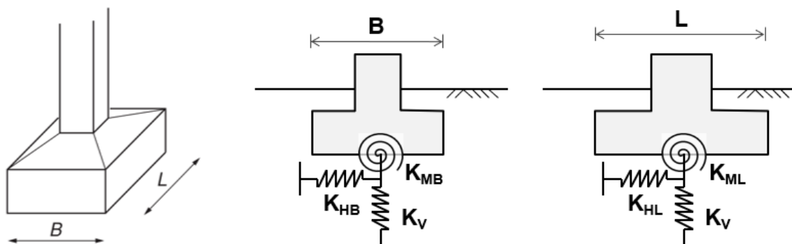
Figure 17 : Raideurs équivalentes pour une fondation isolée
