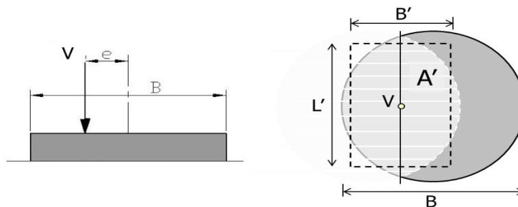
Figure 6 : Définition de l'aire d'assise effective pour une fondation circulaire
