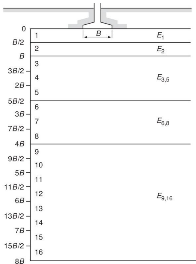
Figure 14 : Modèle pressiométrique pour le calcul des tassements
