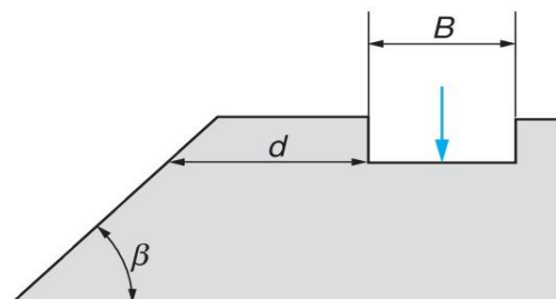
Figure 9 : Présence d'un talus à proximité de la semelle – notations
