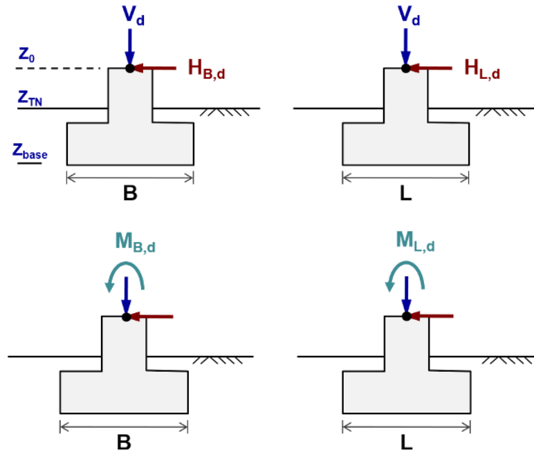
Figure 3 : Conventions de signe dans FONDSUP – Point d’application des charges
