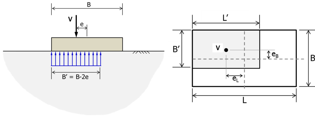
Figure 5 : Définition de l'aire d'assise effective pour une fondation rectangulaire
