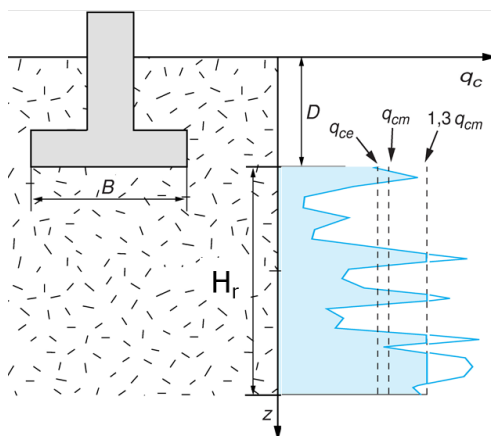
Figure 11 : Principe de calcul de la résistance de cône équivalente (cas d'un traitement par mesures)
