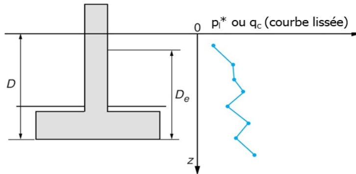
Figure 8 : Notion de profondeur d'encastrement équivalente
