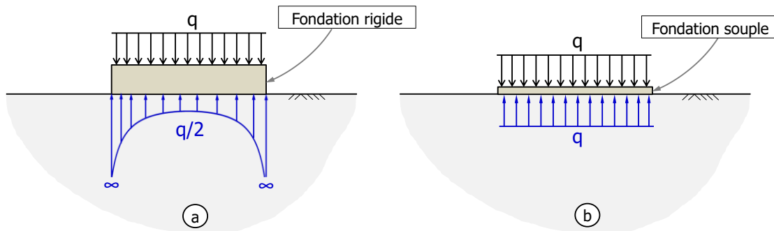
Figure 16 : Distribution des contraintes sous une fondation rigide ou souple (Frank et al. 2018)
