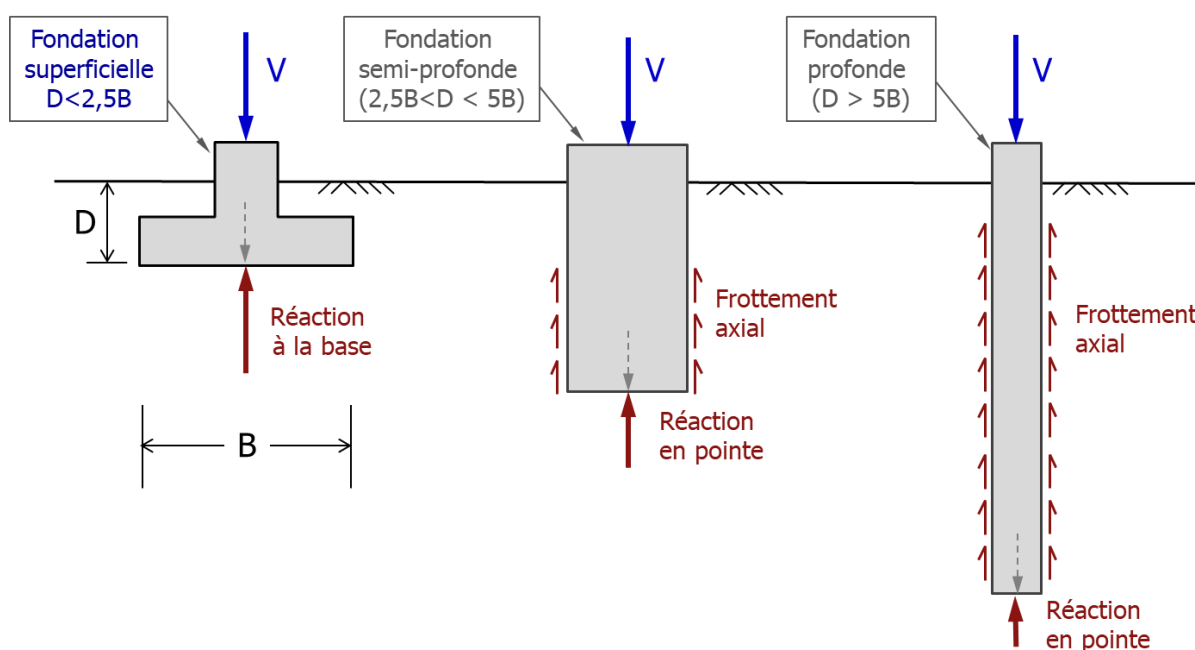
Figure 1 : Domaine conventionnel d'application du concept de fondation superficielle
