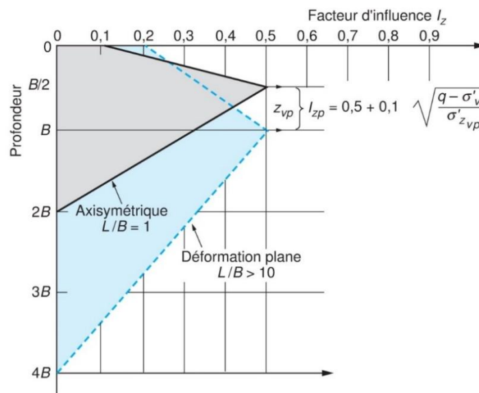
Figure 15 : Facteur d'influence de la déformation verticale
