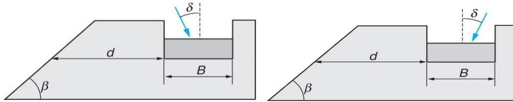
Figure 10 : Proximité d'un talus et charge inclinée – conventions de signe
