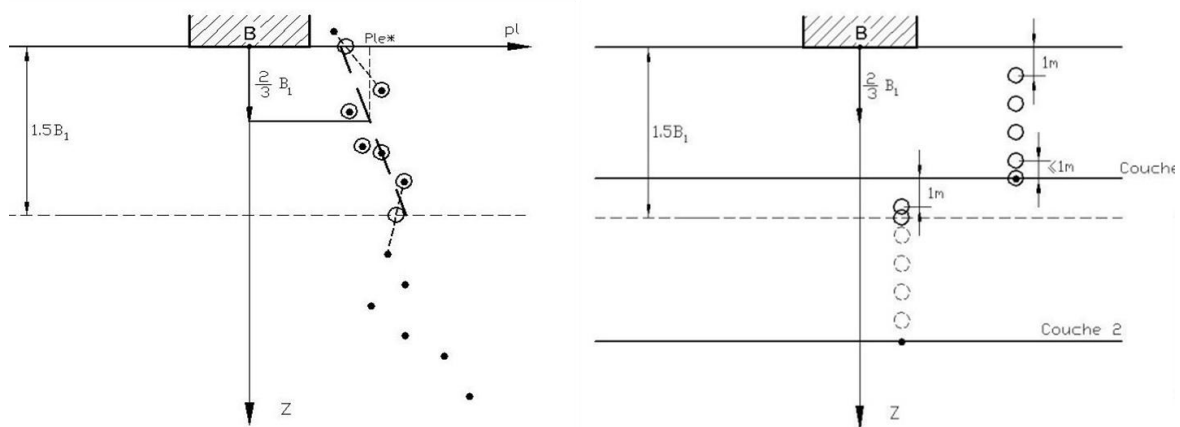
Figure 4 : Différence entre un traitement par mesures (à gauche) et par couches (à droite)
