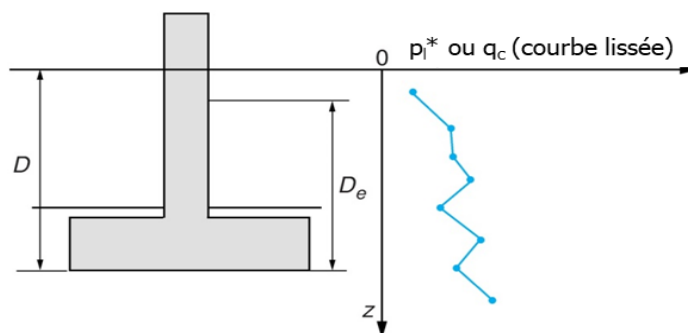
Figure 13 : notion de profondeur d'encastrement équivalente
