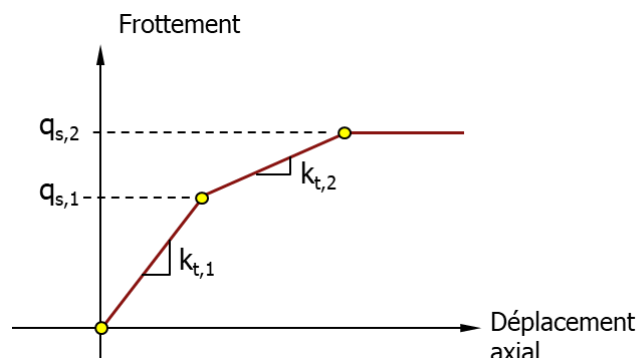
Figure 12 : Courbe de mobilisation à trois paliers – notations et conventions
